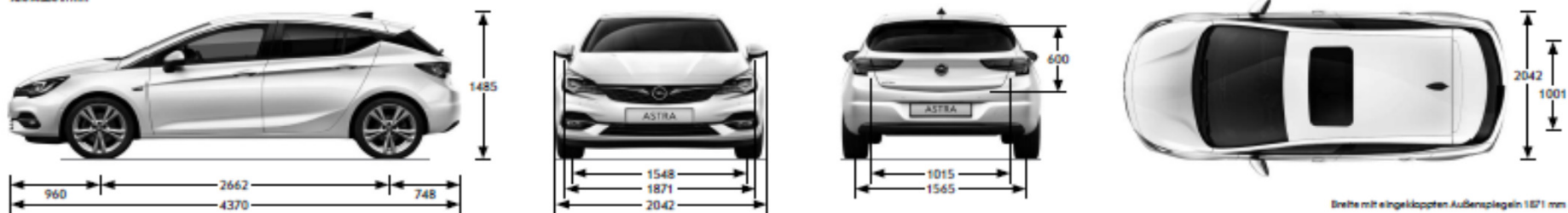
Astra 5-Türer Alle Maße in mm
