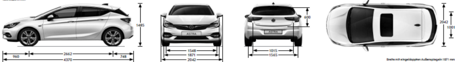
Astra 5-Türer Alle Maße in mm
